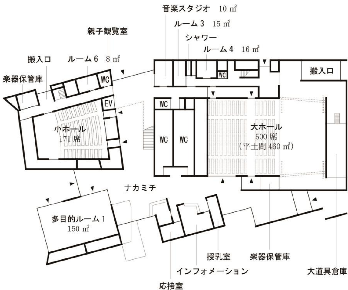
1F 平面図
