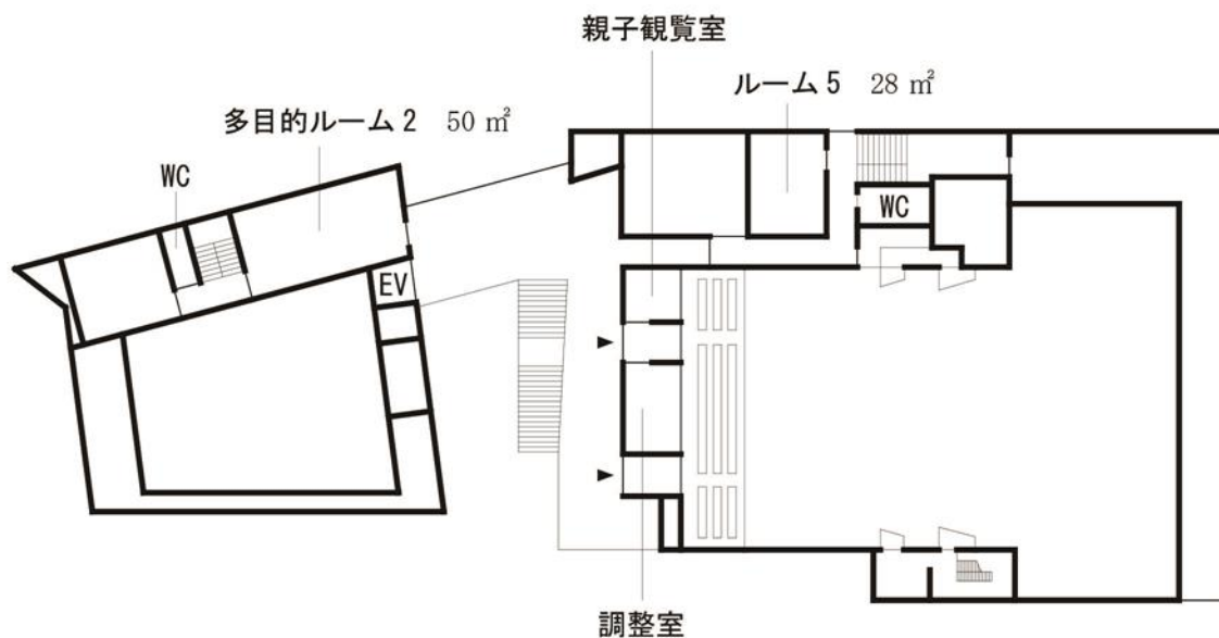
2F 平面図
